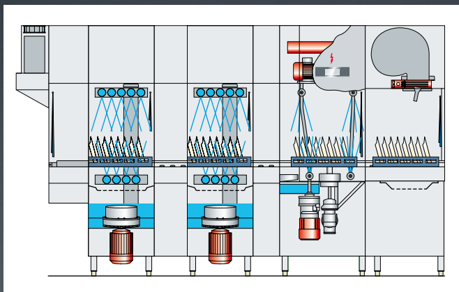
Doorsnede UPster® K-M 280
