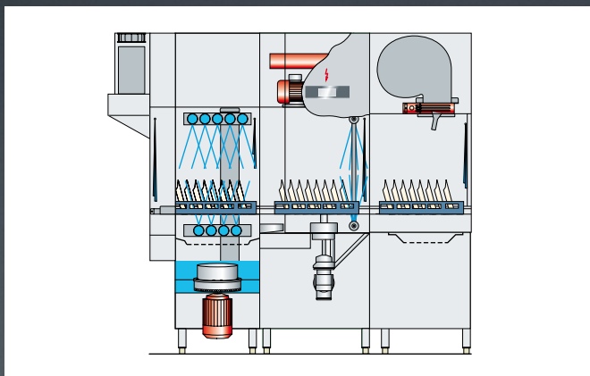
Doorsnede UPster® K-S 160
