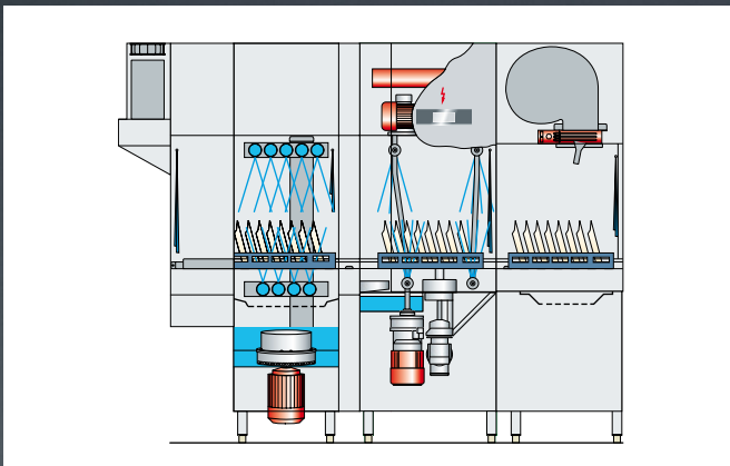
Doorsnede UPster® K-S 200
